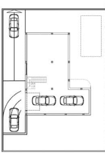
PLANTA SÓTANO
