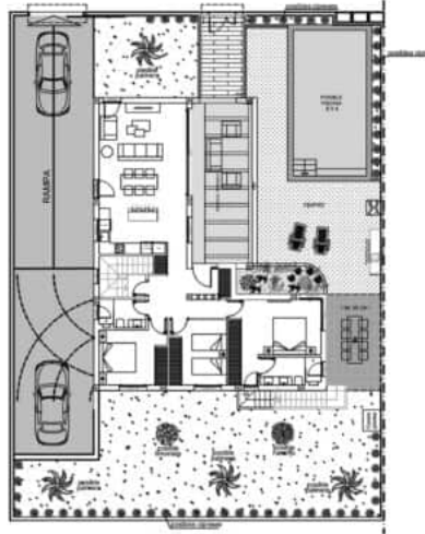
PLANTA BAJA
