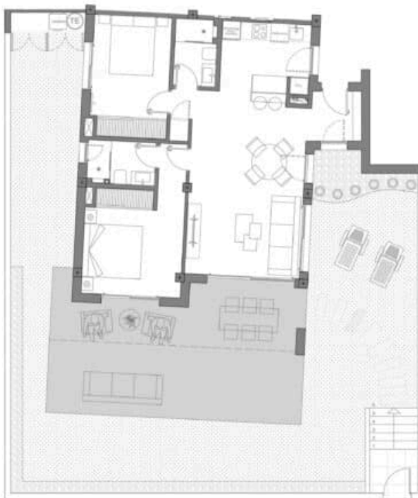
Bloque 3 MODELO ICONIC 2D Nº 17A GARDEN
