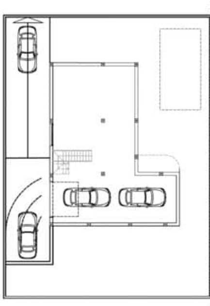
PLANTA SÓTANO
