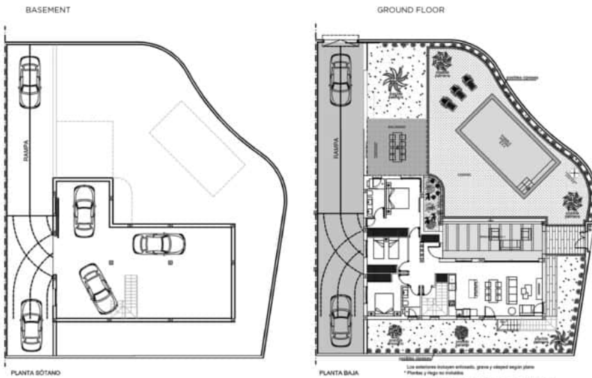
PLANTA SÓTANO
