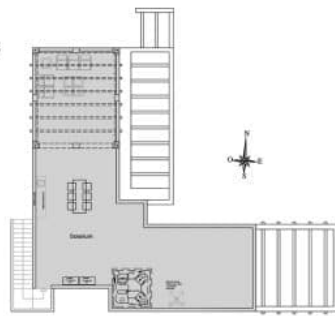
PLANTA SOLARIUM
