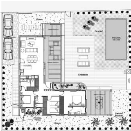
PLANTA BAJA
